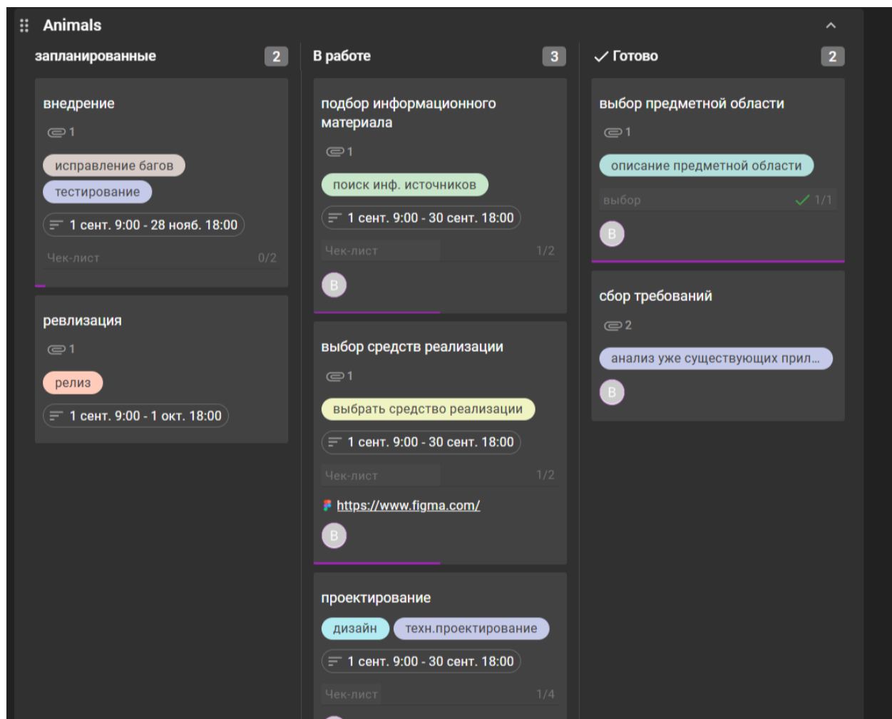
Рисунок 1 – Доска проекта
